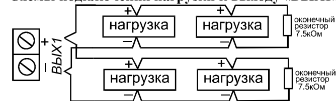
а) двухлучевая схема подключения
