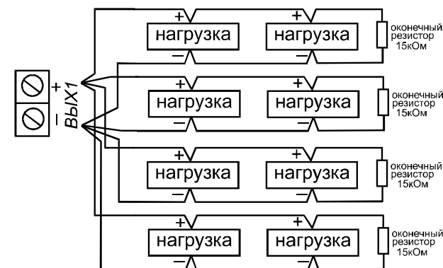
б) четырехлучевая схема подключения
